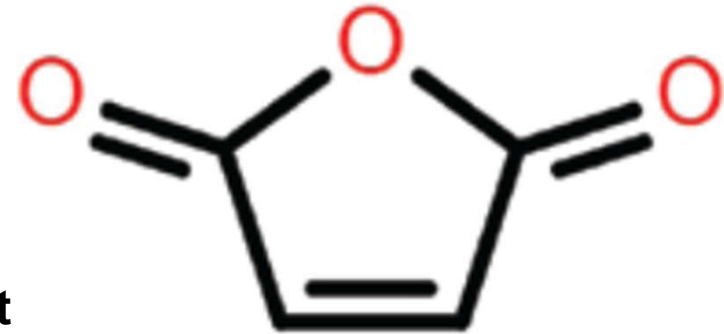
Maleic Anhydride
